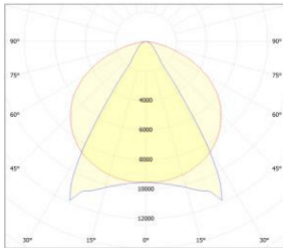
Işık Dağılımı / Light Distribution
