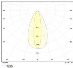
Işık Dağılımı / Light Distribution
